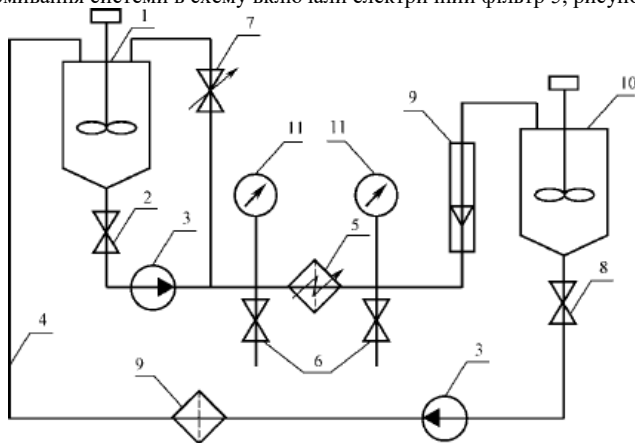
Рис. 1. Схема стенду для визначення повноти відсіювання забрудника:
