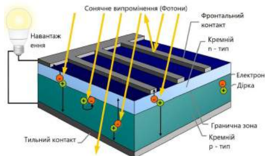
Рис. 1. Структура типової кристалічної кремнієвої фотоелектричної панелі
