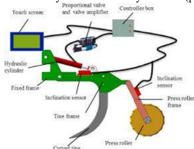
Рис. 2. Електрогідравлічна система керування глибокорихилителем із гнучкими лапами [2]
