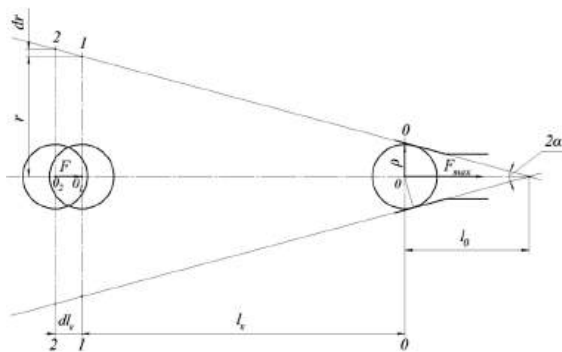
Рис. 1. Схема взаємодії комірки з насінною
