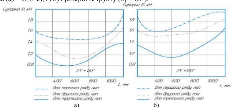
Рис. 3. Залежність значення сумарного тягового опору від відстані розташування розпушувальних лап та кута розкриття ґрунту \Sigma R_x = f(L, 2\gamma)
