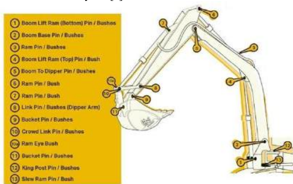
Рис. 1. Типові точки розташування пальців і втулок екскаватора.
