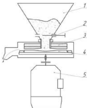
Рис. 1. Схема дискового подрібнювача
