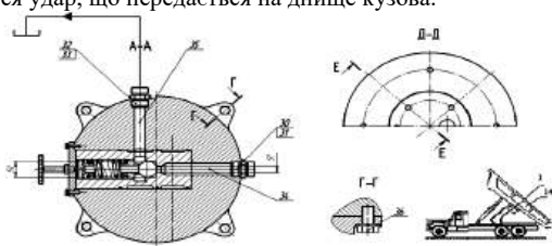
Рис. 4. Конструктивна схема перспективного гідроімпульсного віброударного пристрою для розвантаження кузовів – самоскидів транспортних засобів
