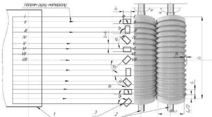
Рис. 2. Розрахунково-технологічна схема подрібнення часіток маси вальцевим подрібнювальним апаратом
