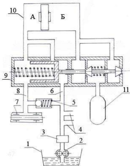
Рис. 1. Схема системи мащення з гідроакумулятором і пневморозподільником:
