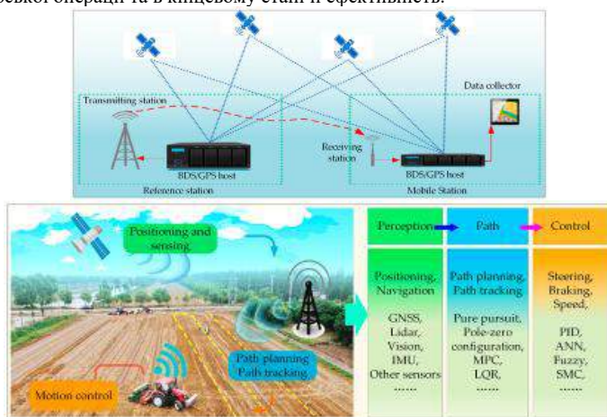
Рис. 1. Принцип дії позиціонування та технології авто навігації [1]
