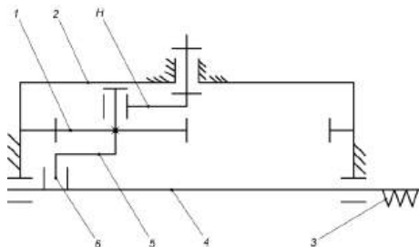
Рис. 2. Схема планетарного механізму приводу різального апарату, з прямолінійним рухом сателіта:
