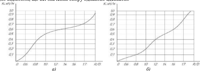
Рис. 1. Залежність питомого тягового опору від співвідношення радіусу сфери до діаметру гладенького диска K_m а - (R/D) , D = 600 \text{ мм} R=800 \text{ мм} і кут атаки \alpha = 22^\circ ; б - (R/D) , D = 700 \text{ мм} R=630 \text{ мм} і кут атаки \alpha = 22^\circ .
