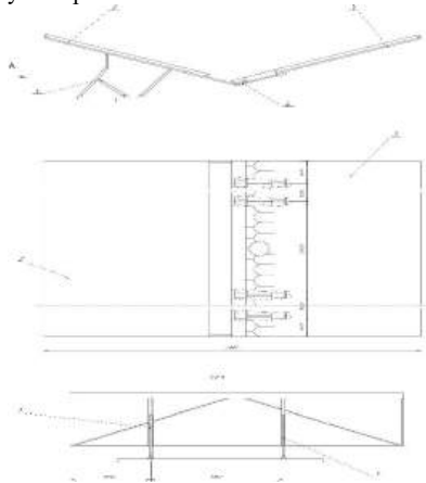
Рис. 2. Вловлювач плодів
