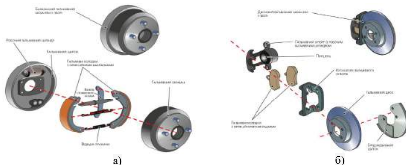
Рис. 2. Приклади гальмівних механізмів: а) барабанний; б) дисковий.
