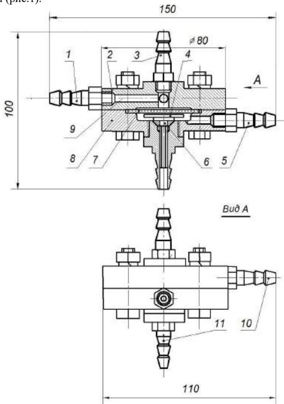
Рис. 1. Сухий затвор для воднево-кисневої зварювальної установки:
