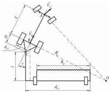
Рис. 4. Схема повороту запропонованого МТА [4]
