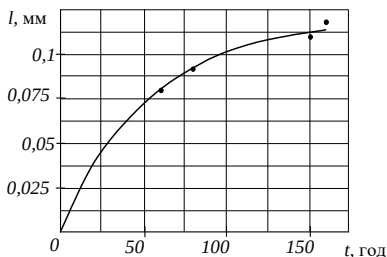
Рис. 1. Залежність деформації повзучості лопатки крильчатки від наробітку
