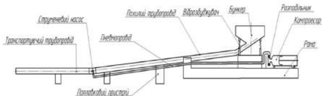
Рис. 1. Схема пневматичного трубопровідного транспортера сапропелів
