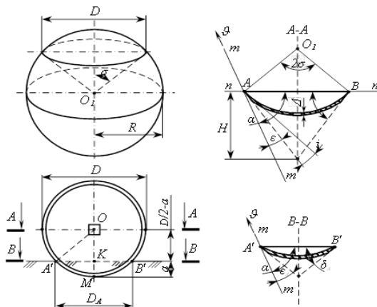
Рис. 1. Схема сферичного диска з основними параметрами
