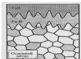
Рис. 1. Будова борованого шару, сформованого за дифузійним механізмом.
