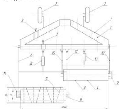
Рис. 1. Комбінований ґрунтообробний агрегат
