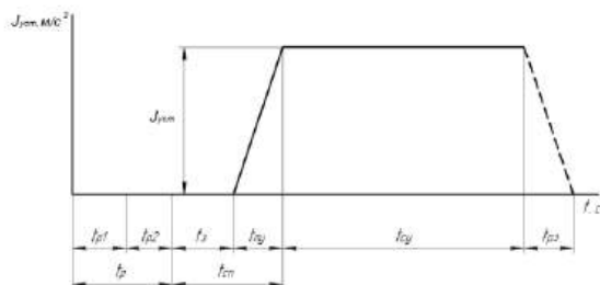
Рис. 1. Гальмівна діаграма автомобіля: t_p – тривалість реакції водія; t_{сп} – тривалість спрацювання гальмівної системи; t_{cy} – тривалість гальмування зі сталим уповільненням; t_{p3} – тривалість розгальмування
