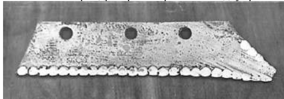
Рис. 2. Точкове покриття леміша плугу. Наробіток - 39 га
