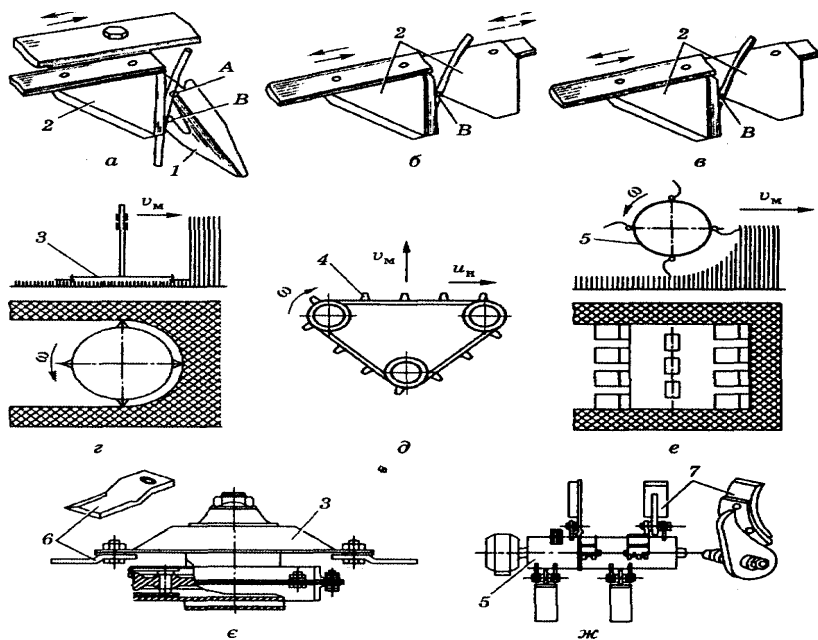
Рис. 2. Схеми найбільш розповсюджених різальних апаратів [8]
