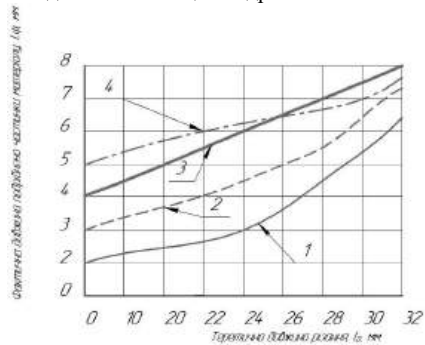
Рис. 4. Графічні залежності впливу фактичної довжини подрібнення маси l_f від теоретично довжини різання l_p при різних кутах входження частинки:
