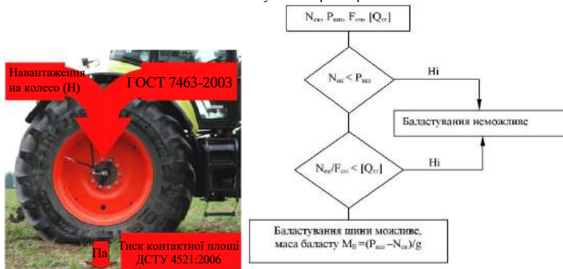
Рис. 4. Обмеження експлуатаційного навантаження на рушій
